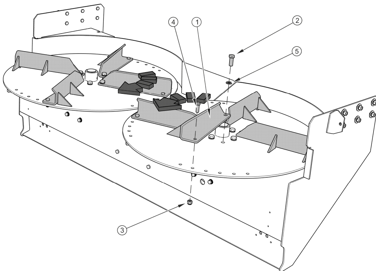
RYСУNEK 5.14 Wymiana łopatek tarczy rozrzucającej
