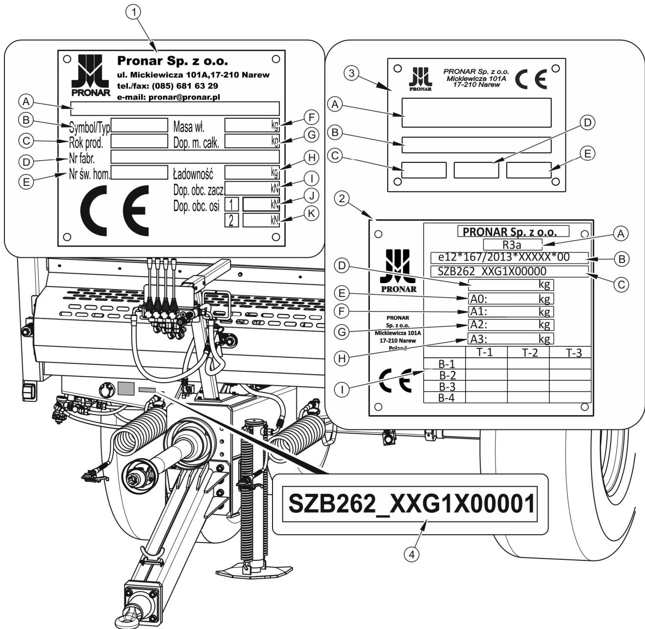
RYСУNEK 1.1 Identyfikacja rozrzućnika
