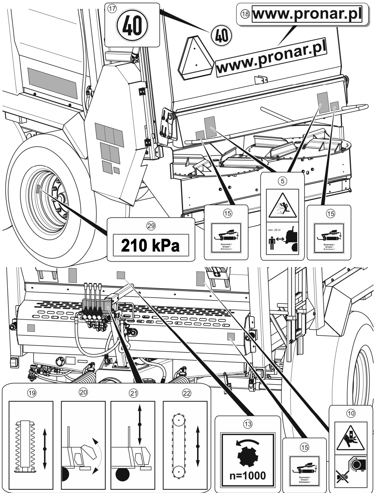
RYSUNEK 2.5 Rozmieszczenie naklejek informacyjnych i ostrzegawczych
