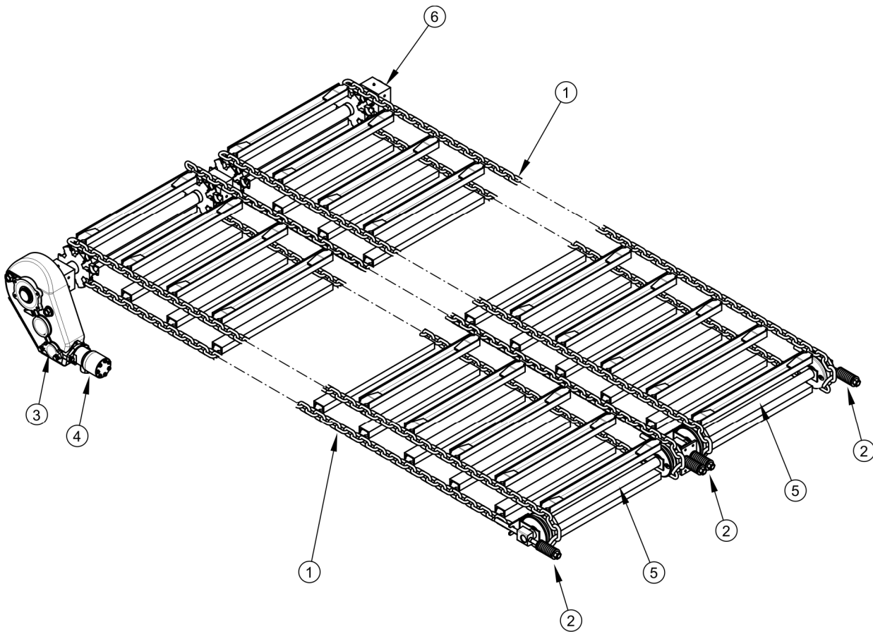
RYСУNEK 3.2 Mechanizm podający
